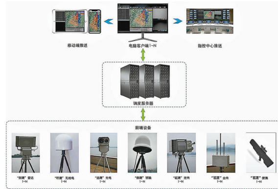
「降鷹」反無人機系統示意圖。受訪者供圖
