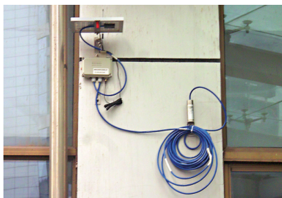
西南醫科大學附屬中醫醫院建築物上的單點無線傳輸採集儀。記者 李兵 攝
