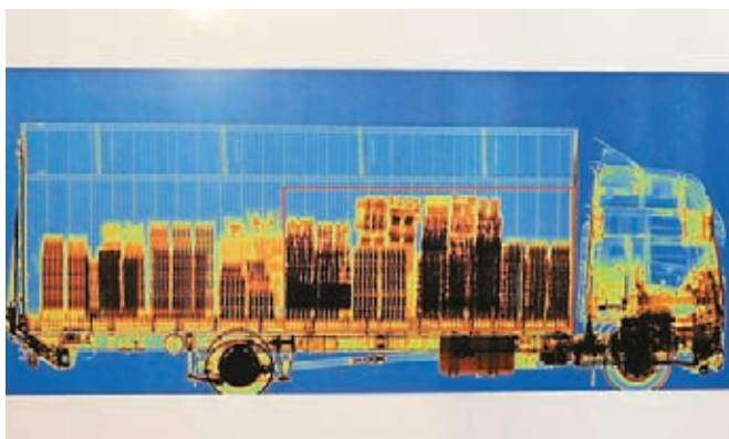
▲用作走私的貨車在X光掃描下,可見貨斗內前後的貨物出現密度差異,紅線內為走私物品。香港文匯報記者劉友光攝
