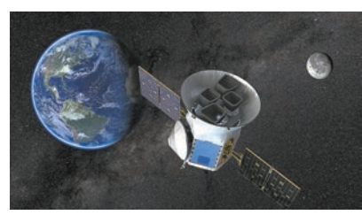
TESS進入軌道後將掃描星體，上為概念圖。 網上圖片
