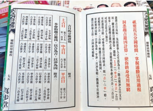
■蔡伯勵的天文曆算《通勝》中的吉日還有上、中、平之分。張岳悅攝
