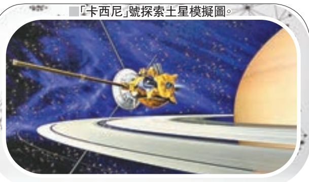
「卡西尼」號探索土星模擬圖。
