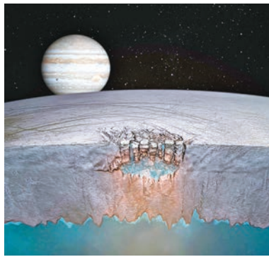
■「木衛二」冰層下存在液態水想像圖。 資料圖片
