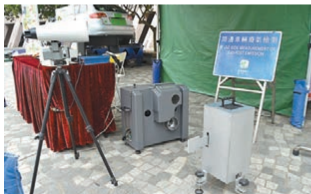
環保署昨日公開展出車輛廢氣測試儀器，加強公眾對空氣質素監測和環保的認識。 羅繼盛 攝
