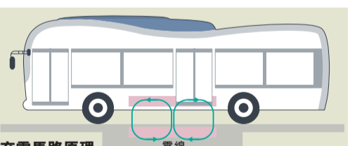
充電馬路原理 ■沿巴士路綫裝設在地底電纜 ■車上的裝置從電磁場吸取電力 ■容許汽車在停下或行駛期間充電 ■電力傳至引擎或儲存於電池
