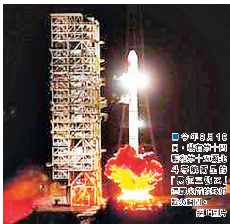
中國北斗衛星導航系統發展歷程 2003年5月發射第三顆北斗衛星 規劃發射5顆靜止軌道和30顆非靜止軌道衛星 2012年建成覆蓋亞太的導航系統 2020年覆蓋全球
