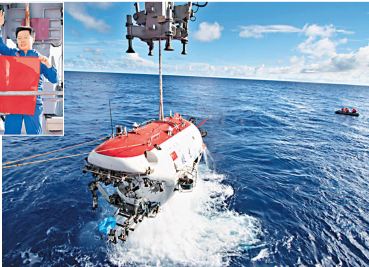
15日，「蛟龍號」在馬里亞納海溝區域的首次下潛試驗中最大下潛深度達6671米，創造中國載人深潛新紀錄。圖為海試結束後，「蛟龍號」出水。
