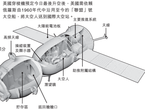
「聯盟」號中央部分能載3人，在軌道上，太空人可移前到軌道艙。
